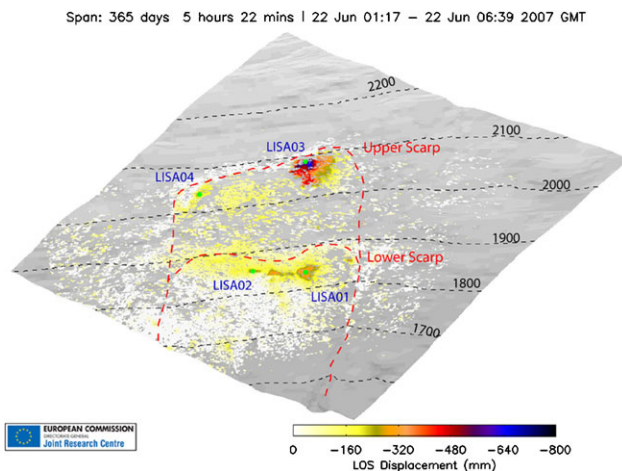
图4 基于4个点（LISA01, LISA02, LISA03, LISA04）的3D累积位移图（2006年6月22日—2007年6月22日）。黑色虚线为等高线，红色虚线为滑坡边界。LOS（line-of-sight）位移的负值表示向观测者的移动距离
